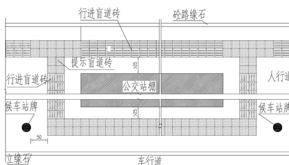
图 4.9.5.2 正规公交站台盲道设置示意图
