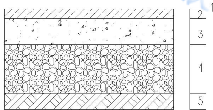
图 4.2.4.3 透水混凝土 I 型结构示意图
