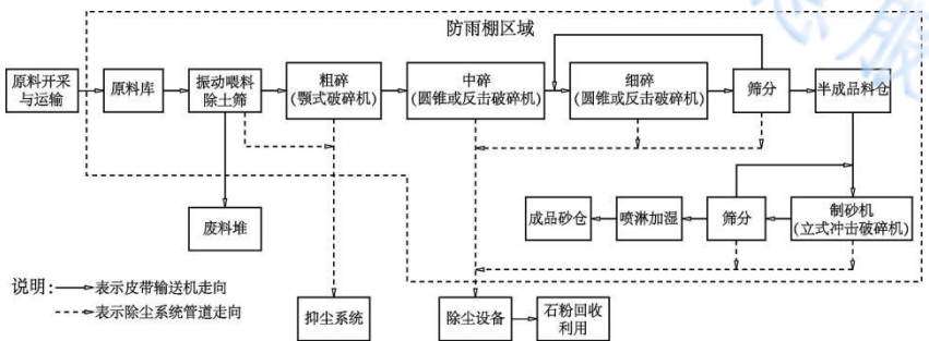
图 A.2.3-1 干法制砂生产工艺流程
