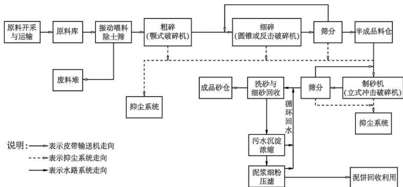
图 A.2.3-2 湿法制砂生产工艺流程
